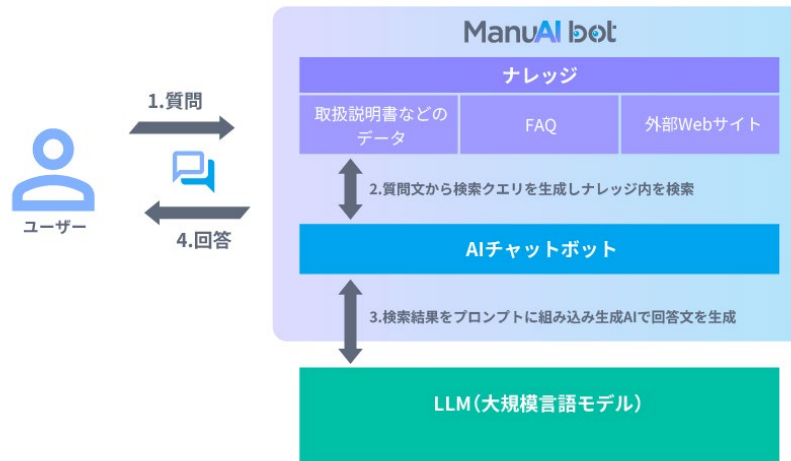
AI チャットボットの技術を支える RAG の仕組み
